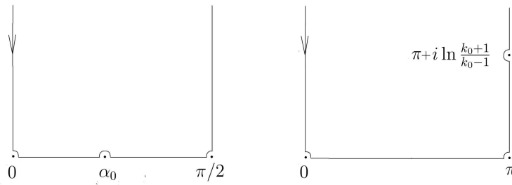
Рис. 4. Конформные свойства l_0 .
