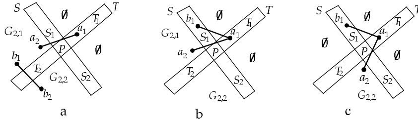
Рис. 2. Разбиение графа парой зависимых разрезов.
